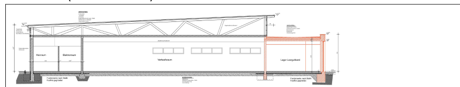
Schnitt A-A (unmaßstäblich)
