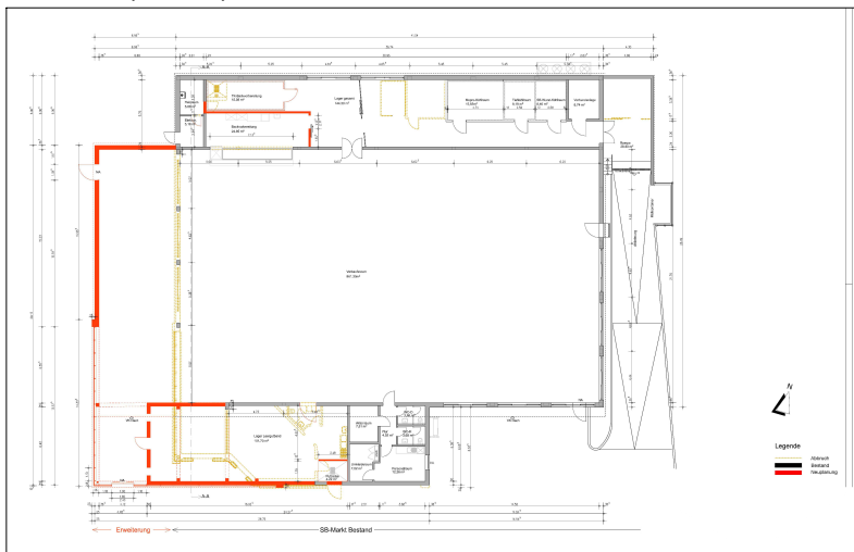
Grundriss (M 1:20)
