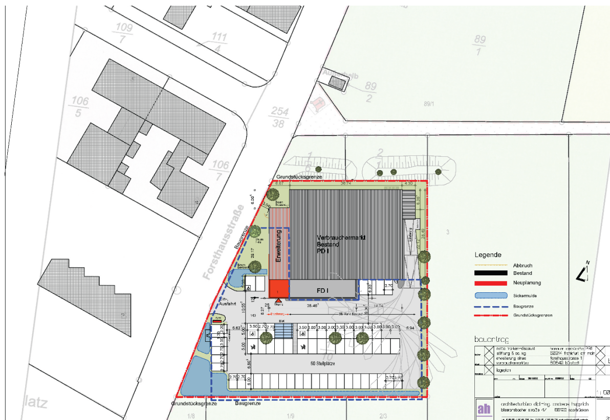
Abbildung 1: Lageplan Nettomarkt mit baulicher Erweiterung (unmaßstäblich)
